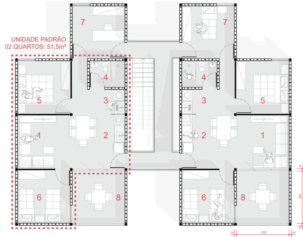
UNIDADE PADRÃO 02 QUARTOS: 51,5m²
