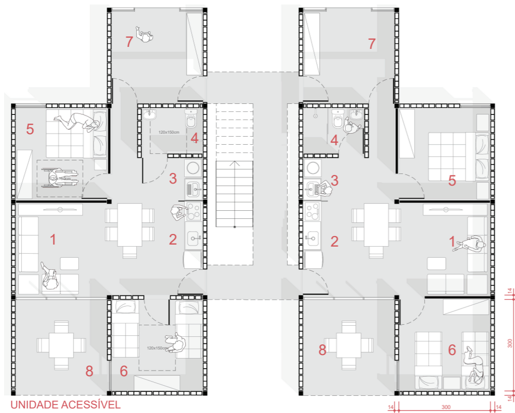
PLANTA PAVIMENTO TÉRREO | ESC. 1:125
